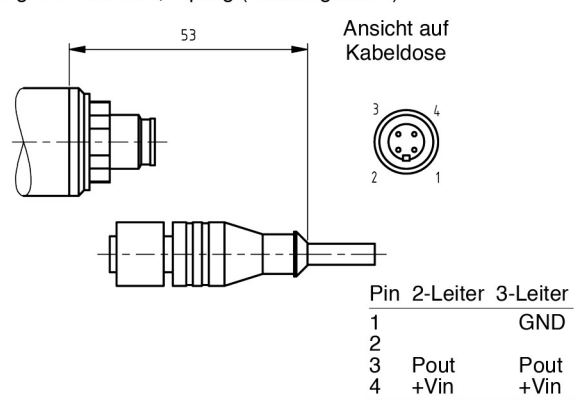
Fig. 15 - M12 x 1, 4-polig (Lumberg RSF4)
