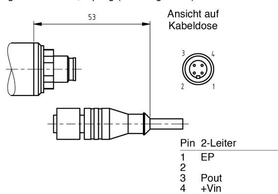
Fig. 15 - M12 x 1, 4-polig (Lumberg RSF4)
