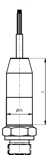
Fig. 10 mit Anschlussgewinde
