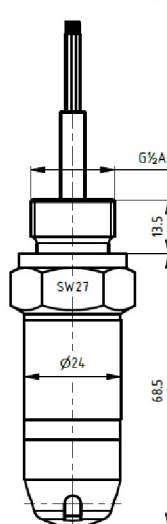
Fig. 11 mit G 1/2 A Rohrverschraubung
